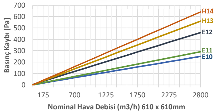
HEPAFIL MN
