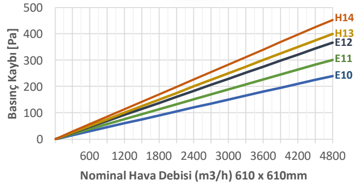
HEPAFIL MF
