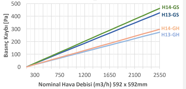
HEPA_AS GS-T
