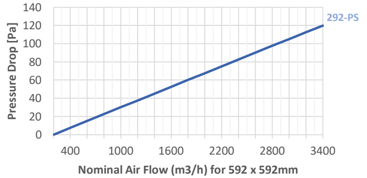
RIGIBAG PS
